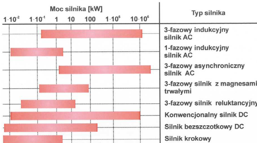
Rys. 1. Zakresy mocy uzyskiwanych przez różne konstrukcje silników elektrycznych [1]
