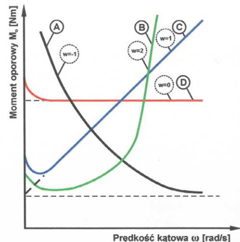
Rys. 2. Charakterystyki mechaniczne maszyn roboczych [1, 3, 4]
